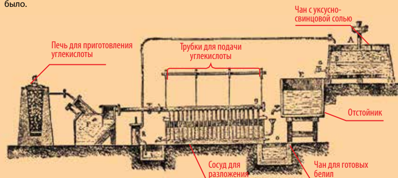
Прибор, используемый для приготовления свинцовых белил по французскому способу
