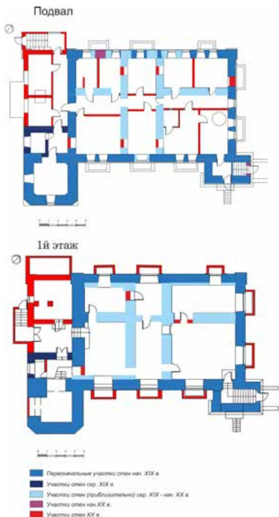
Илл. 6. Схемы строительных периодов стен
