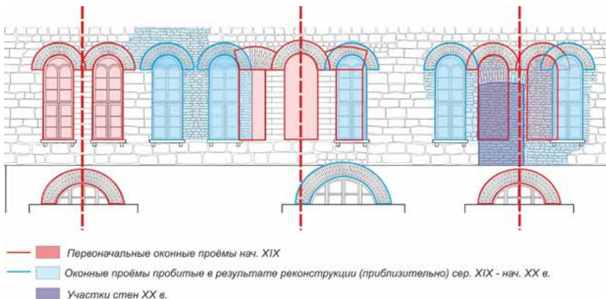
Илл. 4. Анализ строительных периодов западного фасада
