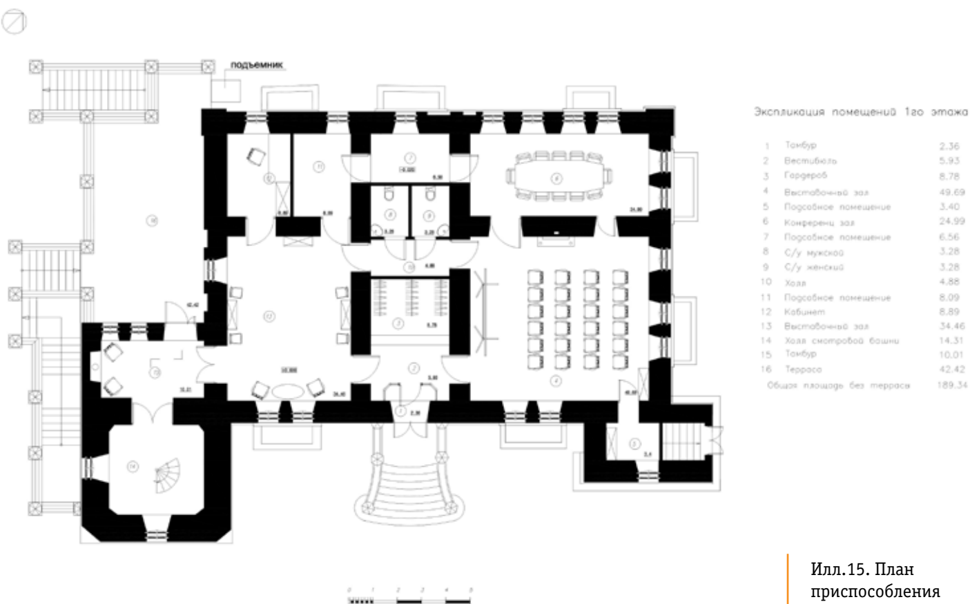
Илл.14. План приспособления цокольного этажа
